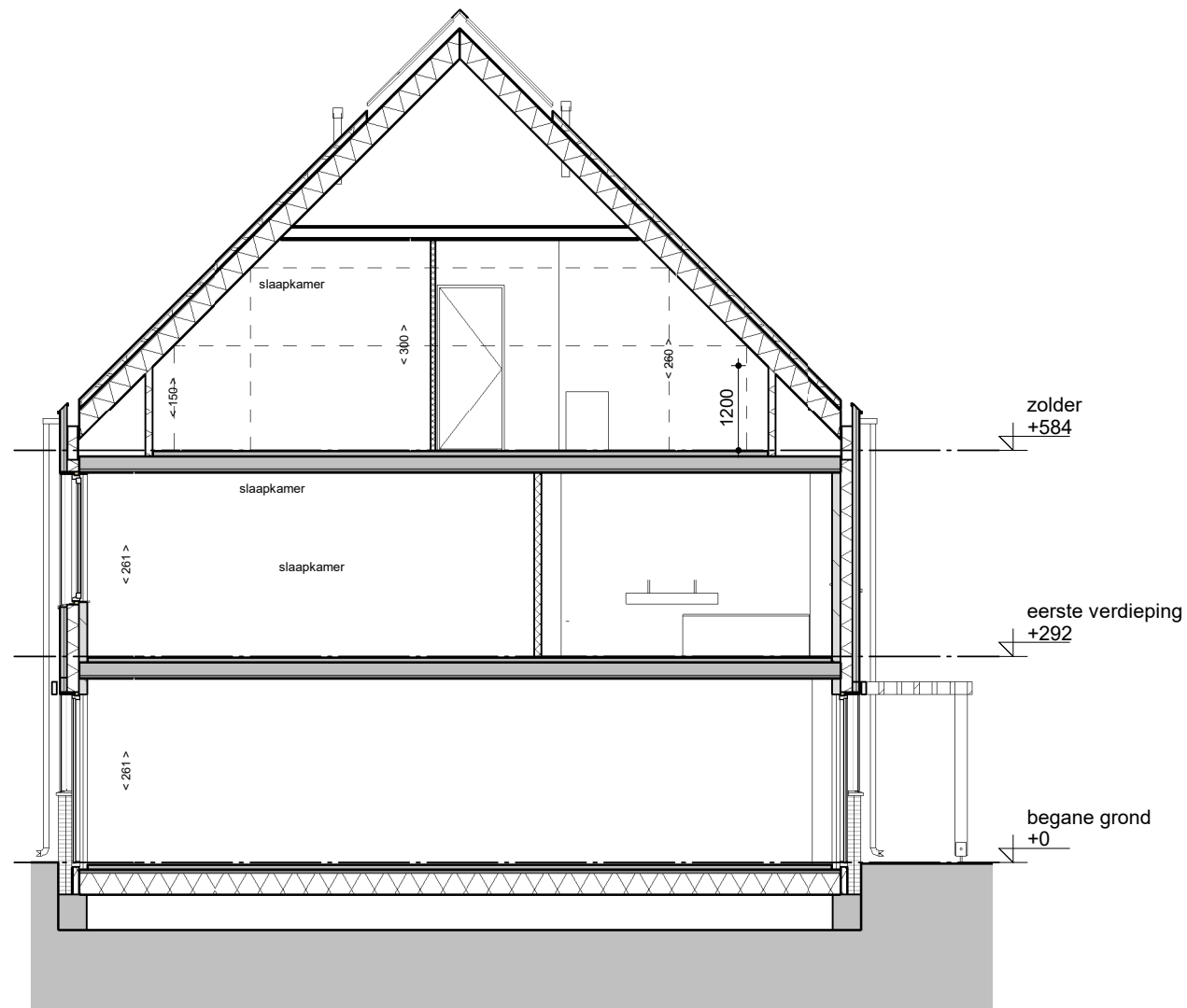
langsdoorsnede
