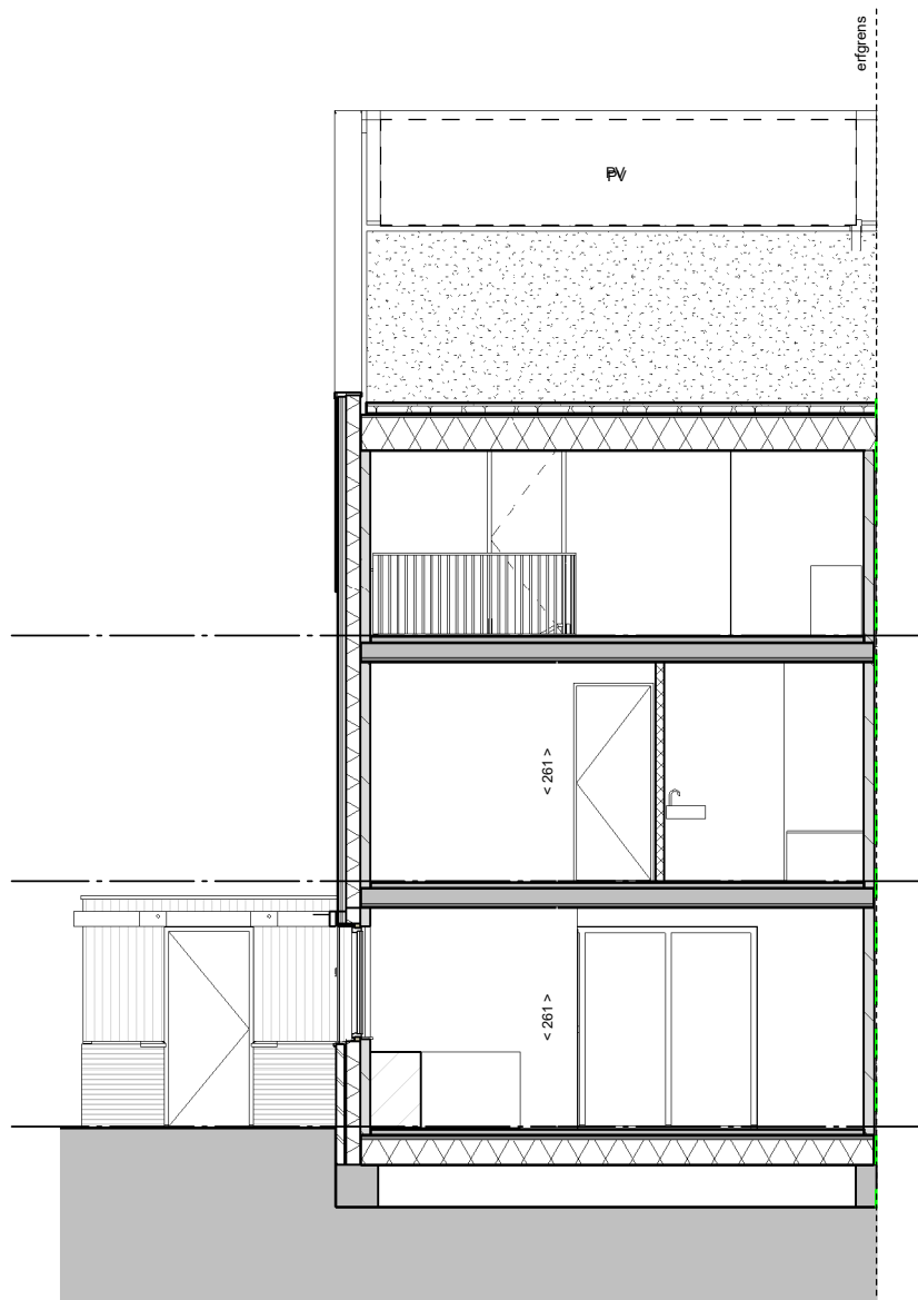
dwarsdoorsnede
